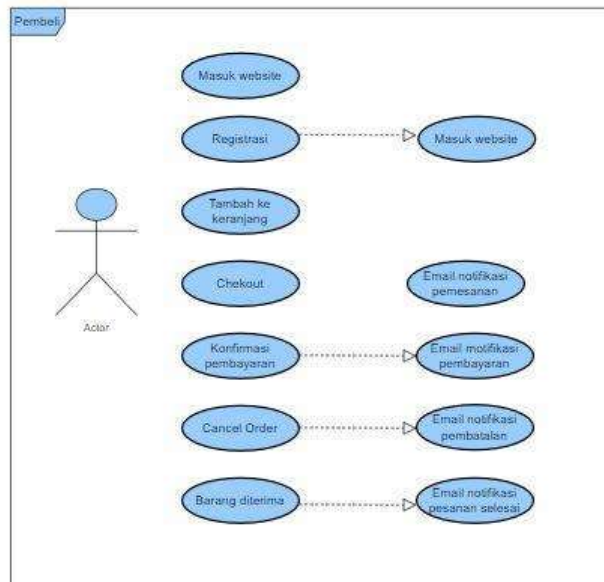
Gambar 3.3 Use Case Diagram Pembeli
