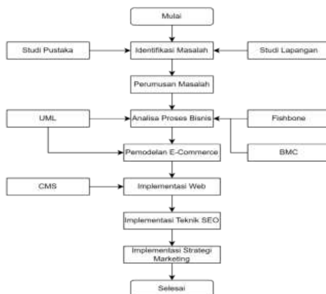
Gambar 2.1 Tahapan Penelitian
