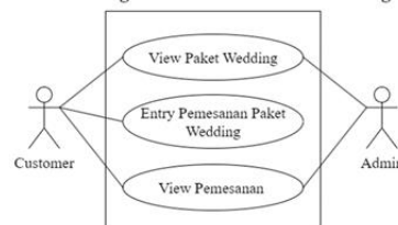
Gambar 4. Use Case Diagram Pemesanan Paket Wedding
