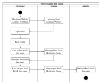
Gambar 9. Activity Diagram Kritik dan Saran
