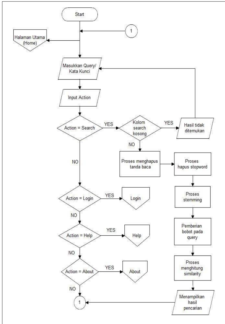
Gambar 2. Flowchart Menu Utama
