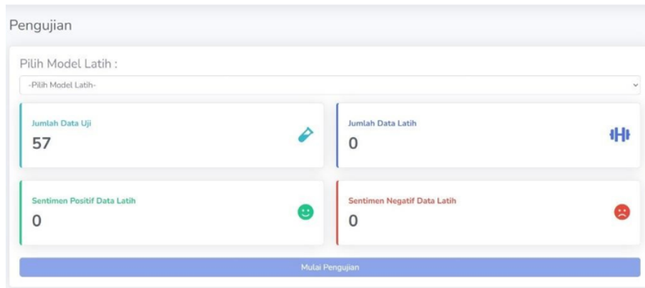
Gambar 7. Pengujian Model
