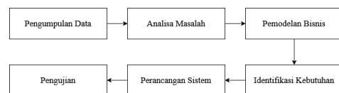
Gambar 1. Tahapan Penelitian
