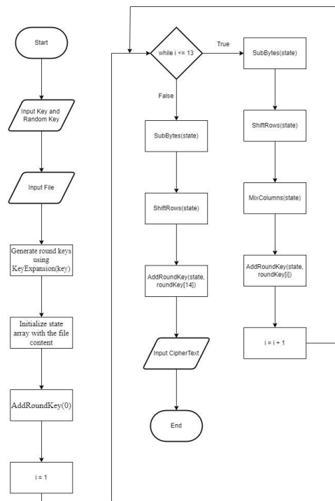
Gambar 4 Flowchart Tahapan Enkripsi
