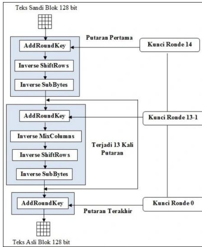
Gambar 3 Tahapan Dekripsi
