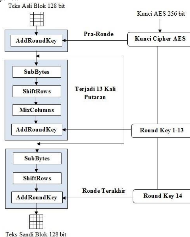
Gambar 2 Tahapan Enkripsi
