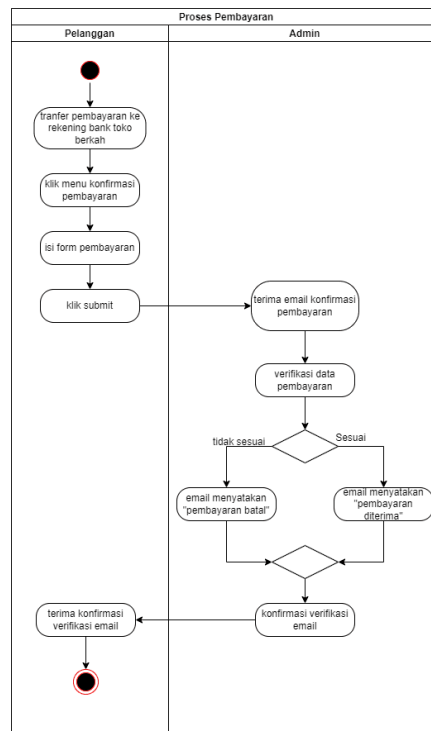
Gambar 5. Activity Diagram Sistem Usulan Proses Pembayaran
