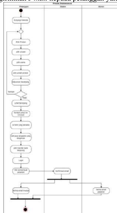
Gambar 4. Activity Diagram Sistem Usulan Proses Pemesanan
