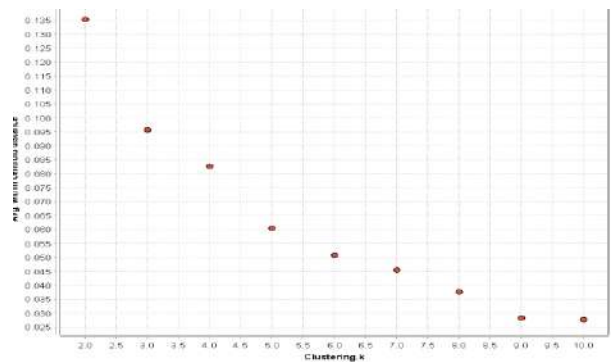
Gambar 9. Grafik Scatter
