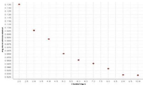
Gambar 11. Grafik Scatter
