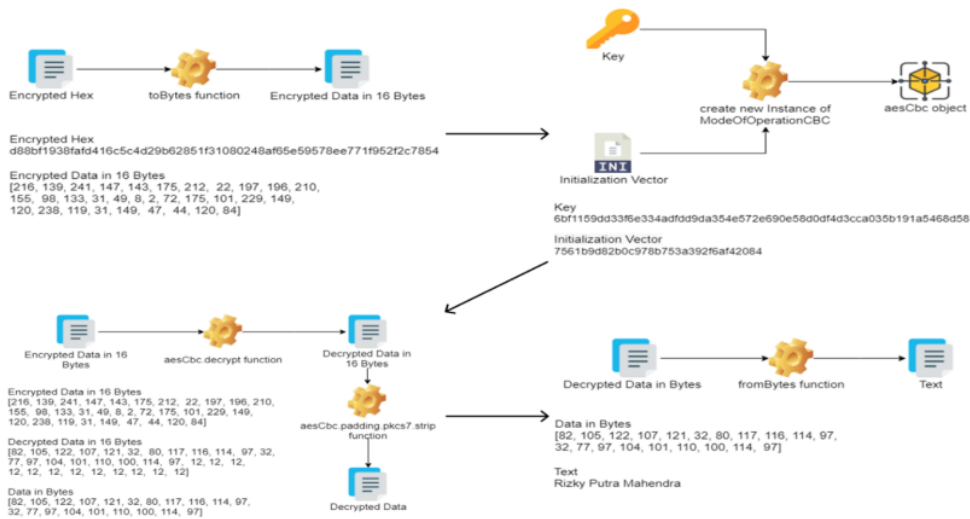
Gambar 8. Proses dekripsi dengan library Aes-js
