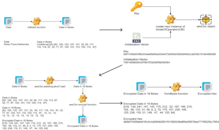
Gambar 7. Proses enkripsi dengan library Aes-js
