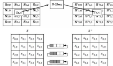
Gambar 3. ShiftRows
