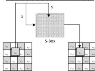
Gambar 2. SubBytes
