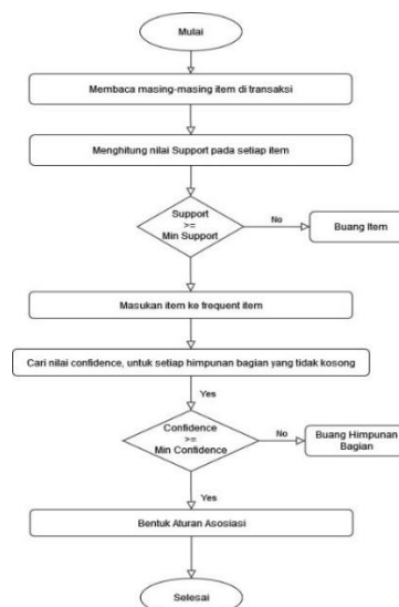
Gambar 3. Flowchart Apriori
