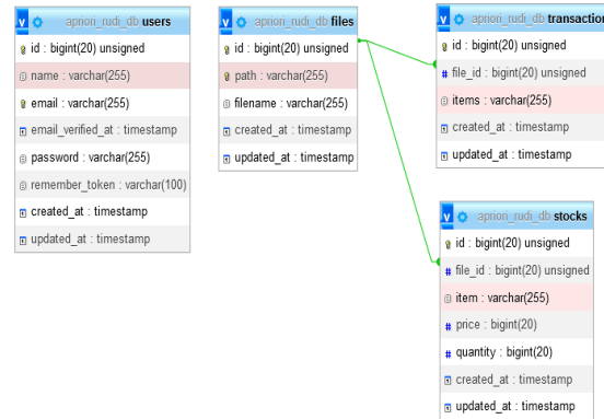
Gambar 2. Rancangan LRS
