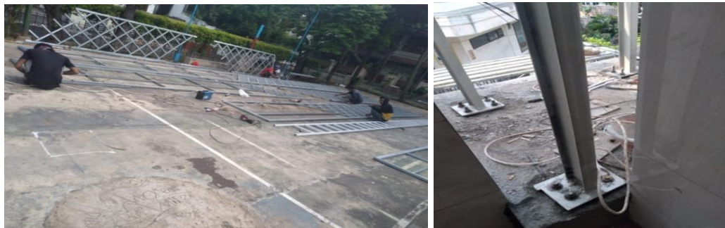
Gambar 8. (a) Fabrikasi Rangka Selubung Minaret (ACP). (B) Ereksi Rangka Utama Minaret.
