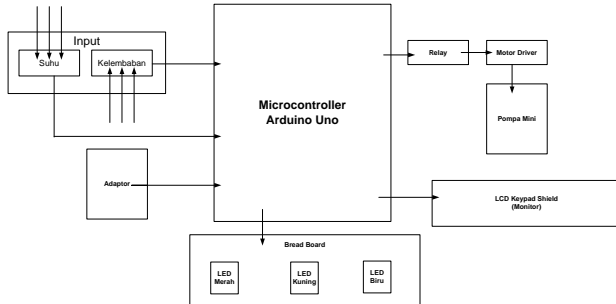
Gambar 3.13 Rangkaian Komponen Modul 2
