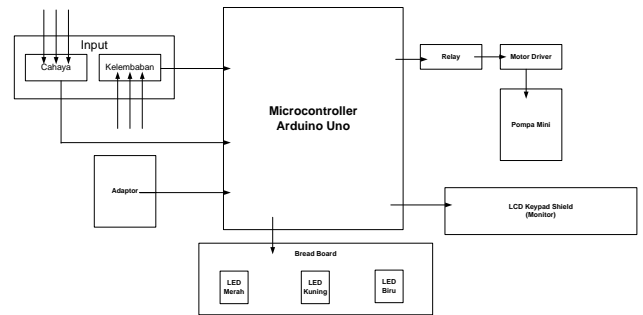
Gambar 3.12 Rangkaian Komponen Modul 1
