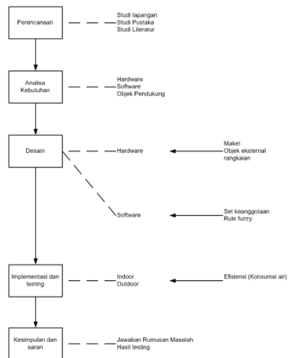
Gambar 3.1 Langkah Penelitian
