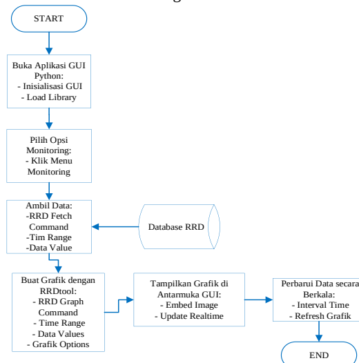
Gambar 13. Tampilkan Data GUI Python
