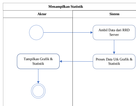
Gambar 7. Activity Diagram Menampilkan Statistik
