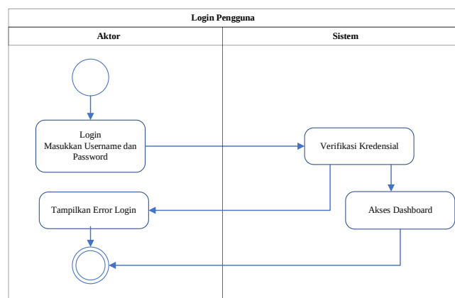
Gambar 4. Activity Diagram Login Pengguna
