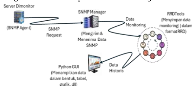
Gambar 2. Rancangan Desain Sistem
