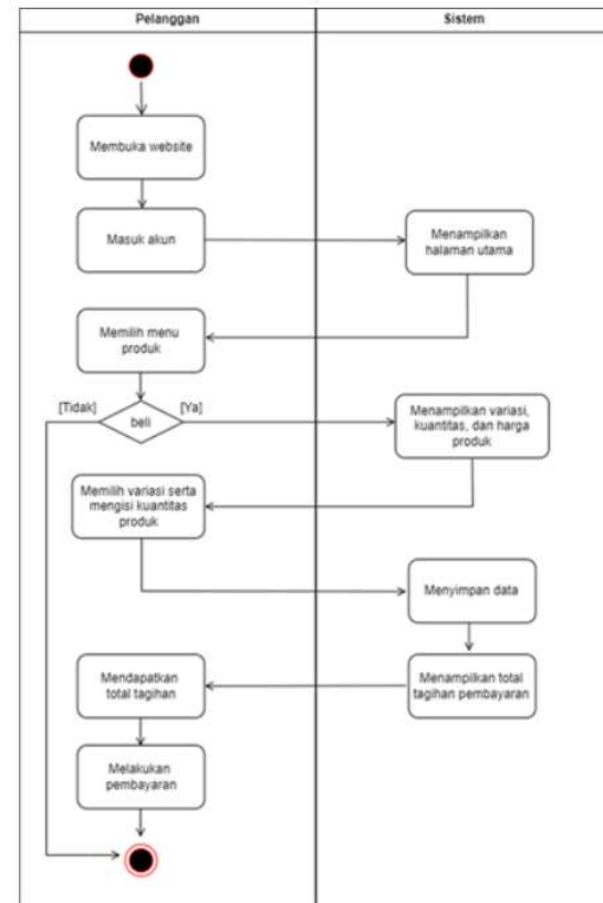
Gambar 8. Activity Diagram Pemesanan Produk
