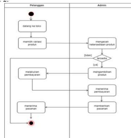
Gambar 2. Activity Diagram Penjualan Produk
