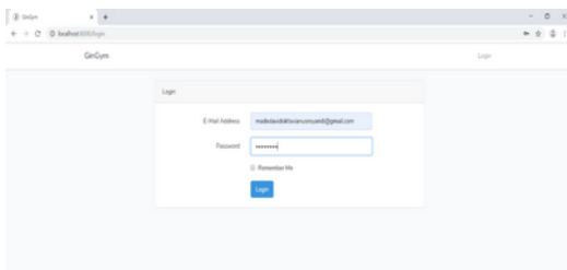
Gambar 6. Login
