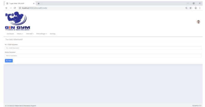
Gambar 8. Tambah Alternatif
