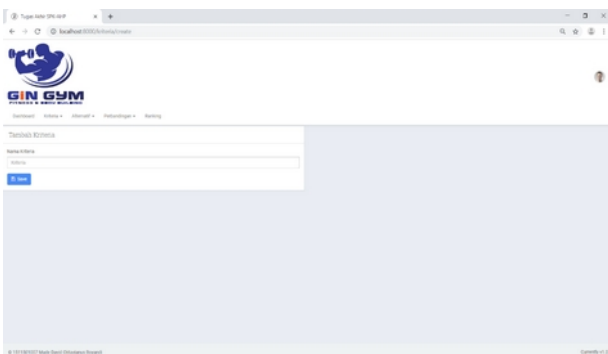
Gambar 7. Tambah Kriteria
