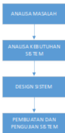
Gambar 1. Langkah-langkah Penelitian
