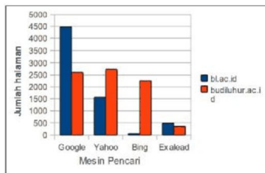
Gambar 2: Perbandingan Size Domain bl.ac.id dan budiluhur.ac.id (Oktober 2010)
