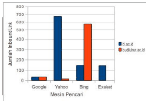
Gambar 1: Perbandingan Visibility Domain bl.ac.id dan budiluhur.ac.id (Oktober 2010)
