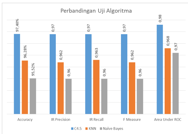
Gambar 1. Perbandingan Uji Algoritma
