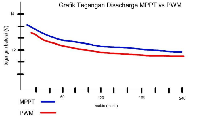
Gambar 7. Grafik Tegangan Discharge
