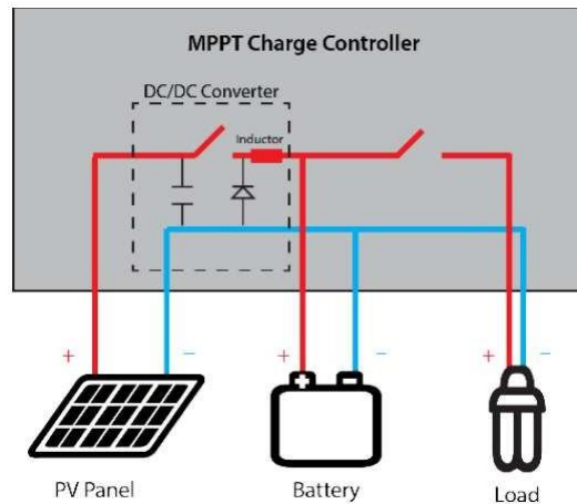
Gambar 3. Sistem Pengendali MPPT
