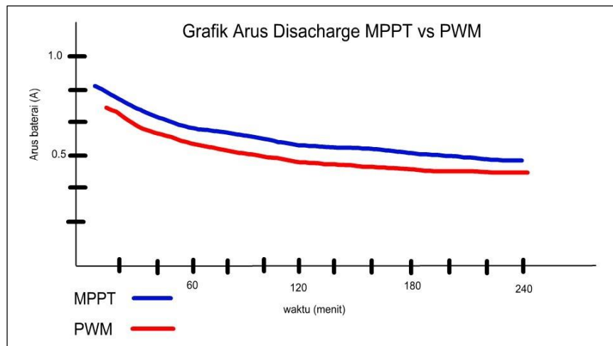
Gambar 8. Grafik Arus Discharge
