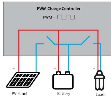
Gambar 1. Sistem dengan PWM
