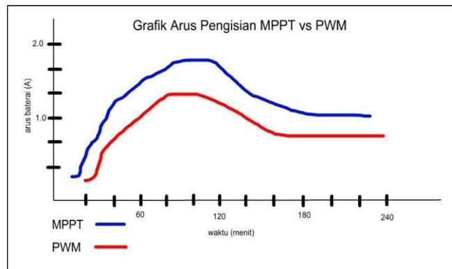
Gambar 6. Grafik Arus Pengisian
